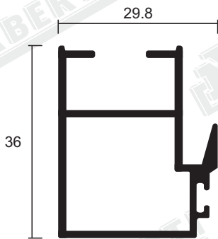
314208- TRASLAPE DE HOJA
