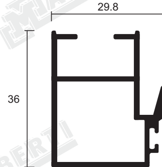
314208-TRASLAPÉ DE HOJA
