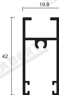
314209-MARCO DE HOJA SUPERIOR
