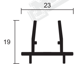
314211-ADAPTADOR DE HOJA
