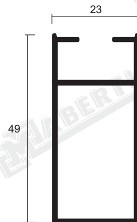
314206-MARCO DE HOJA LATERAL
