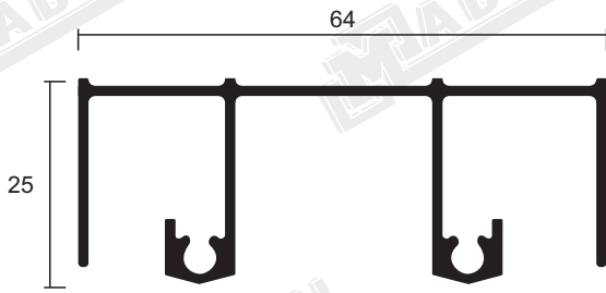
314201-MARCO SUPERIOR
