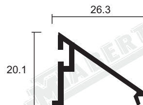
323604-JUNQUILLO
