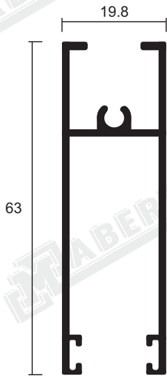
364201- MARCO DE HOJA INFERIOR REFORZADA
