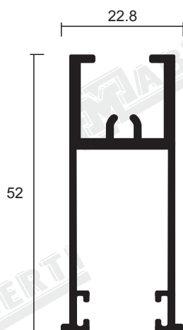
314210-MARCO DE HOJA REFORZADO
