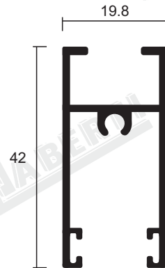
314209- MARCO DE HOJA SUPERIOR
